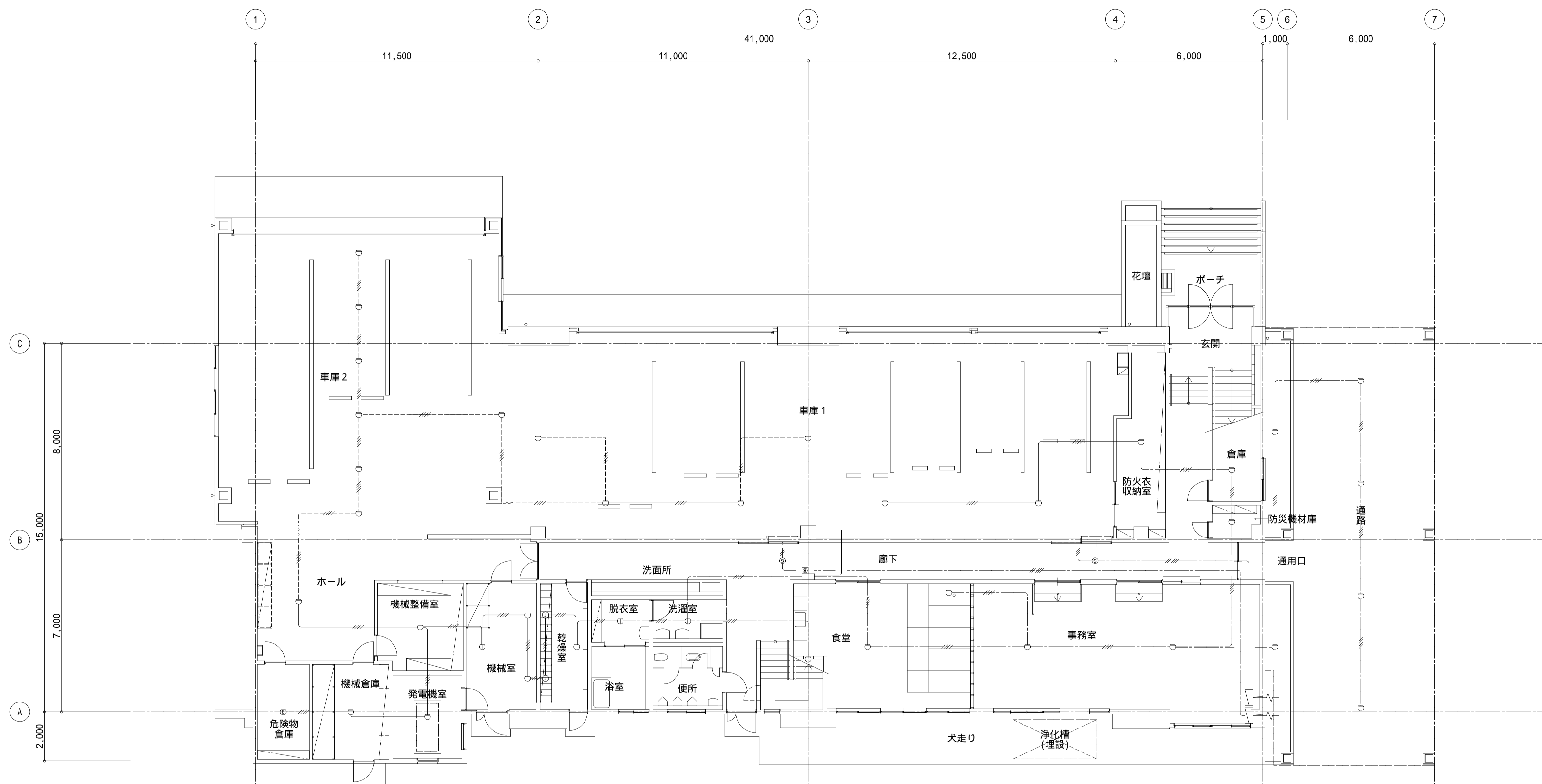
庁舎棟 弱電設備 1 F 平面図 S=1/100
