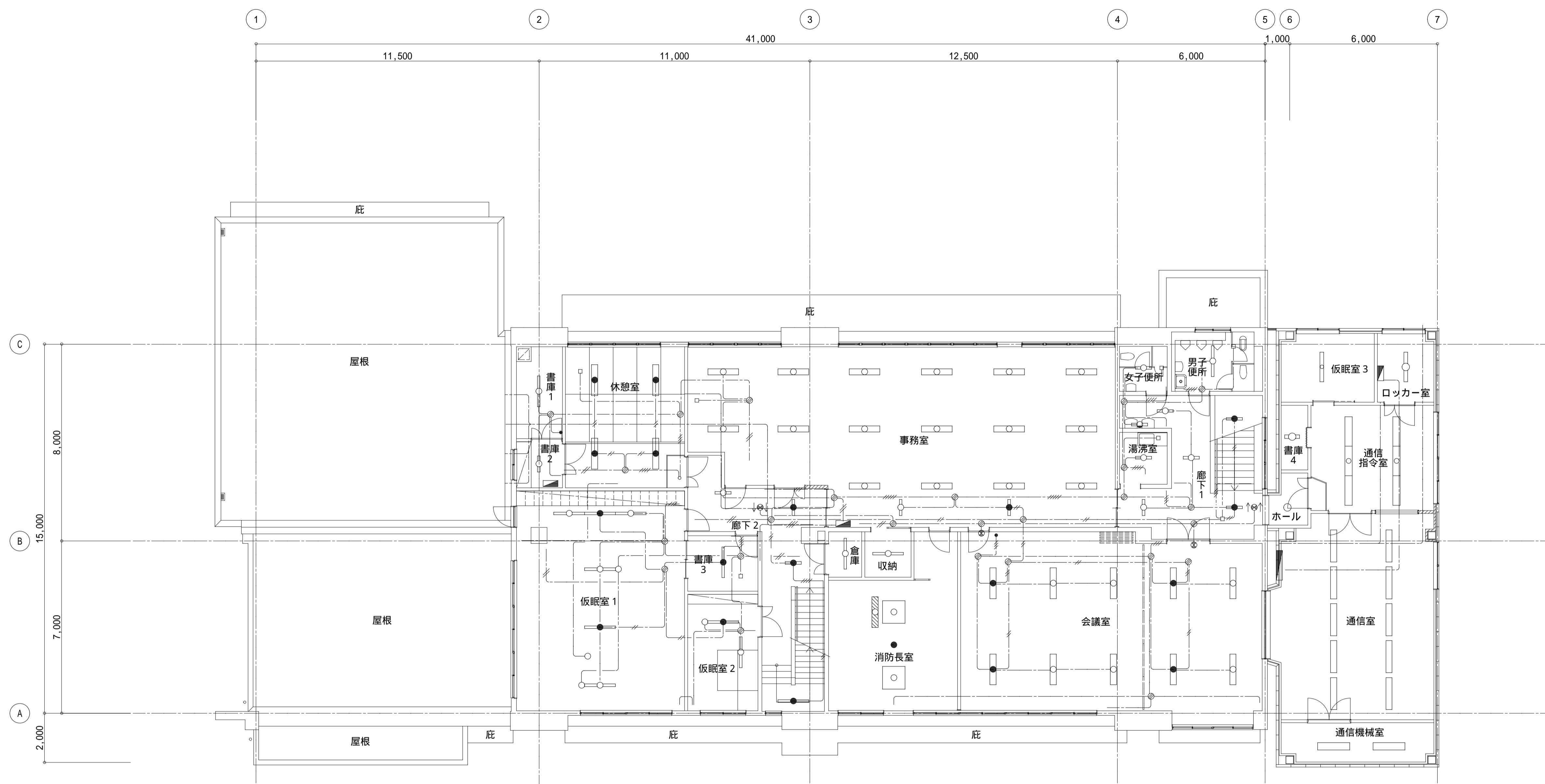
庁舎棟 電灯・幹線設備 2 F 平面図 S=1/100
