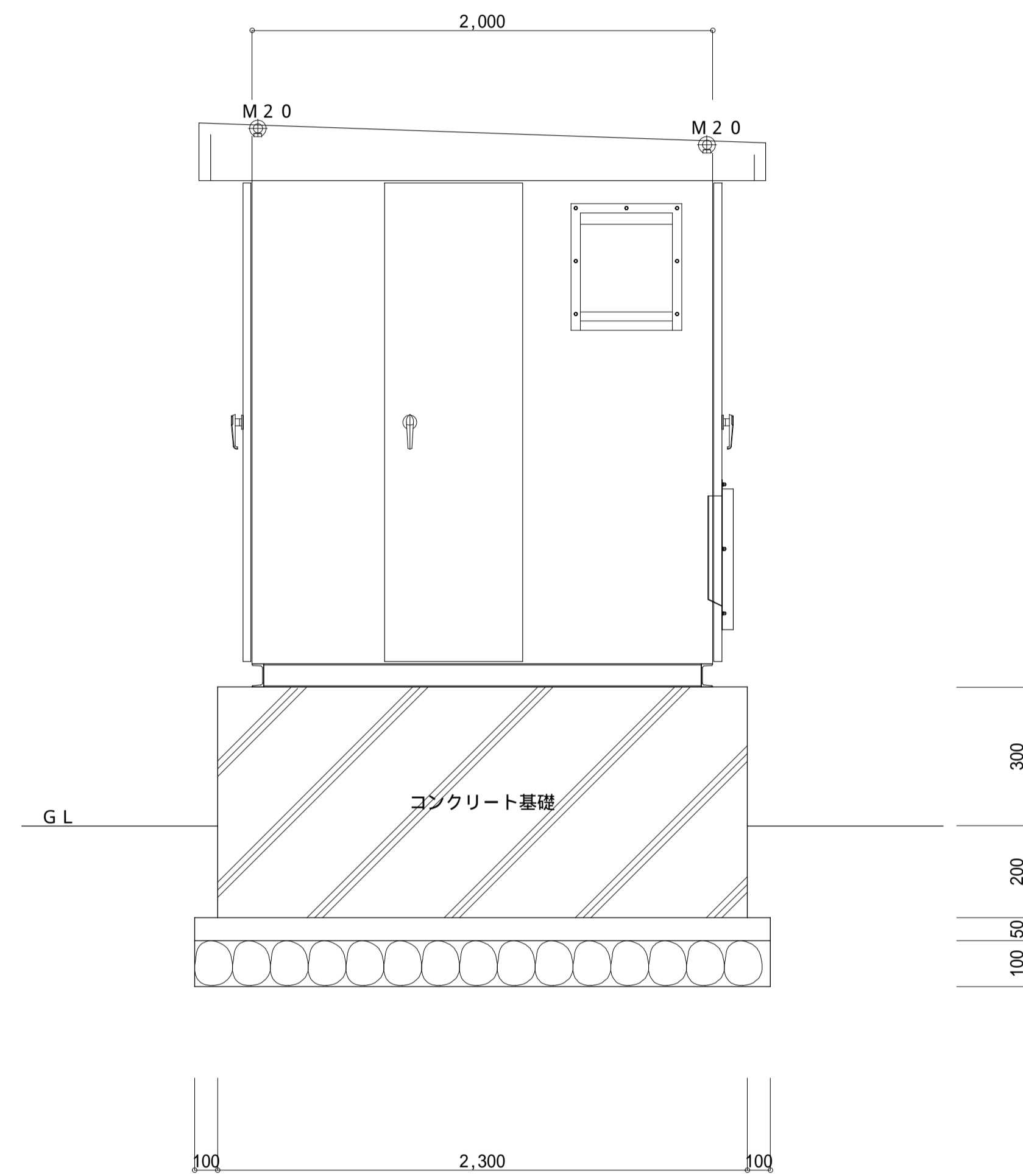
右側面図
