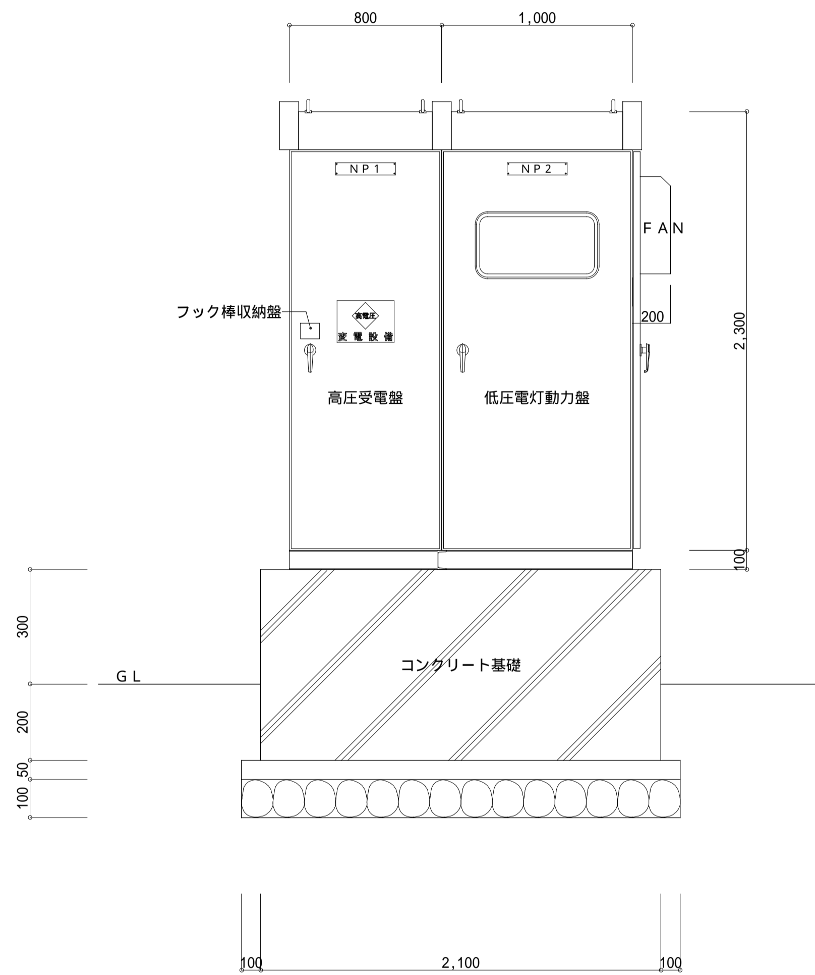
正面図
