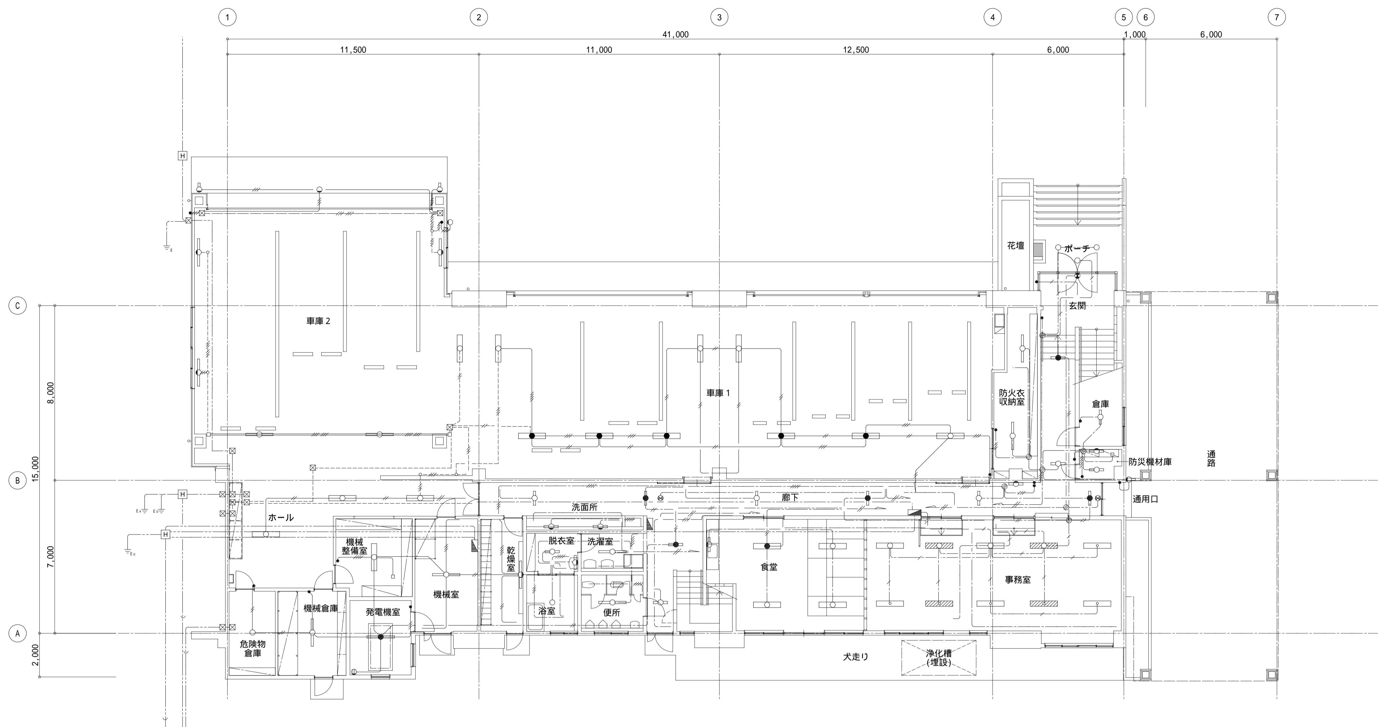
庁舎棟 電灯・幹線設備 1 F 平面図 S=1/100
