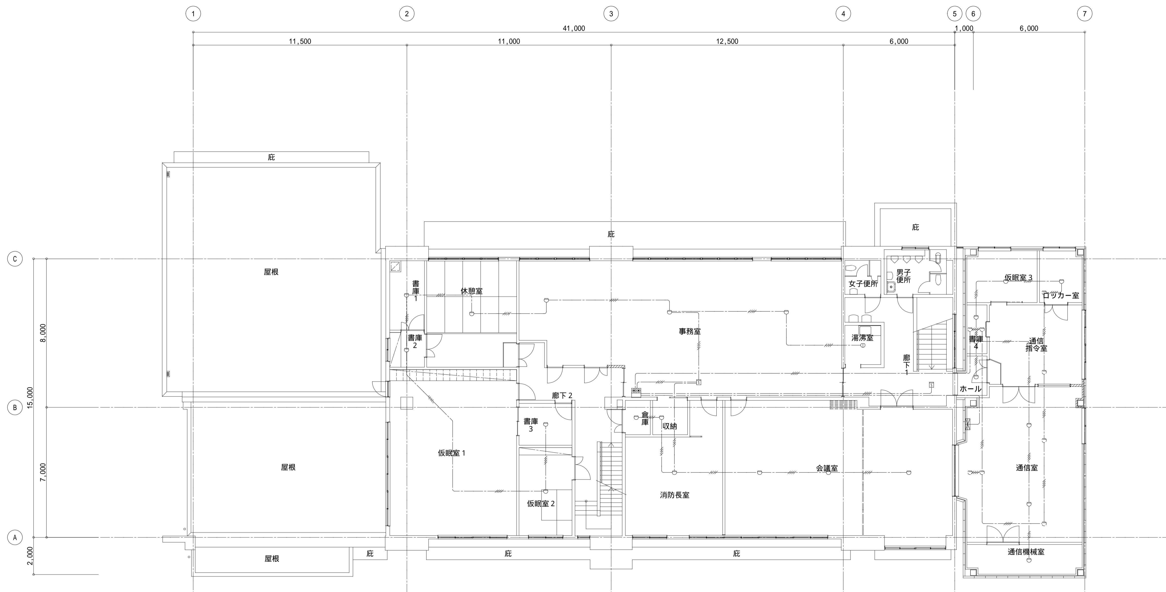
庁舎棟 弱電設備 2 F 平面図 S=1/100
