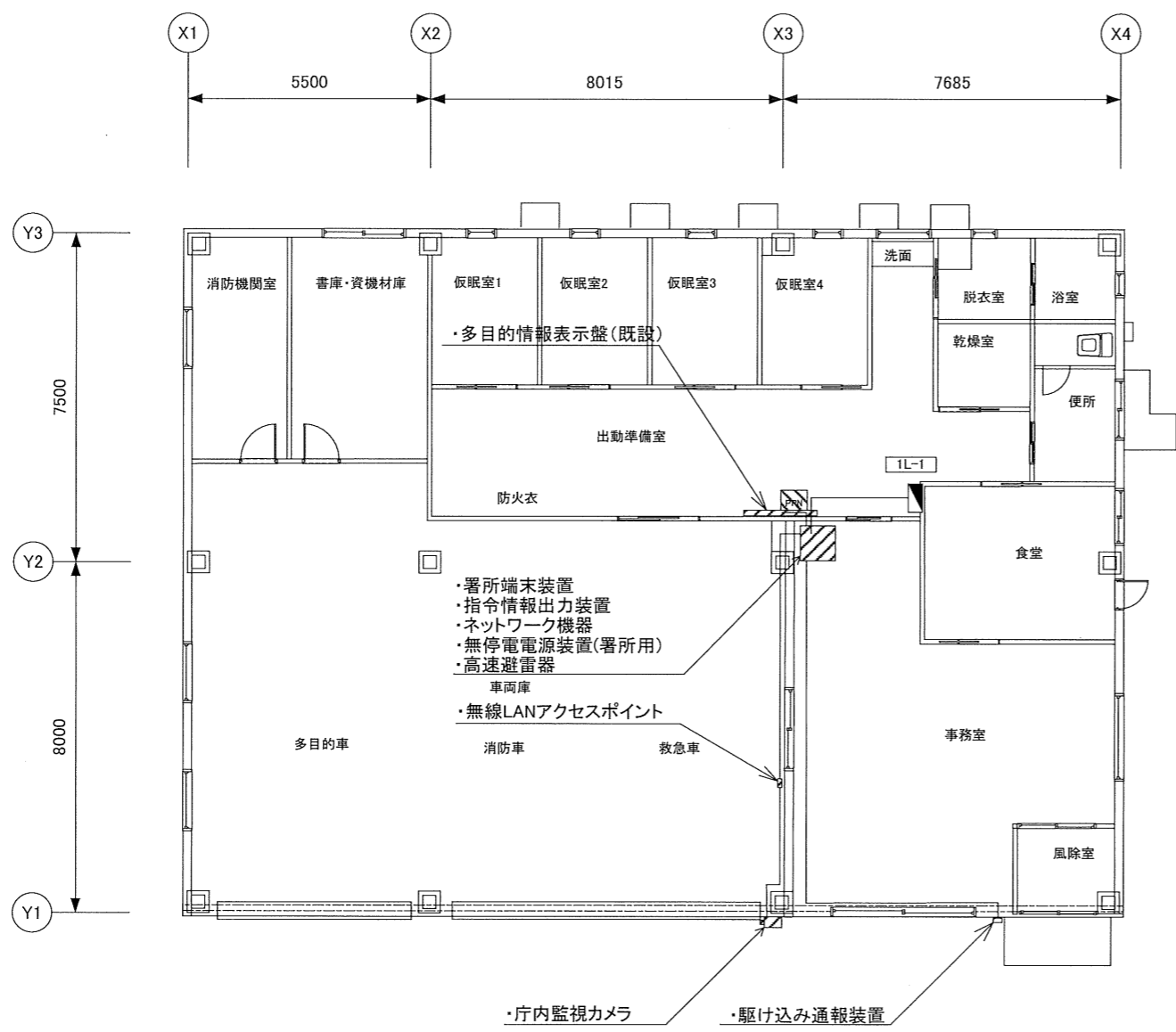
平面図
