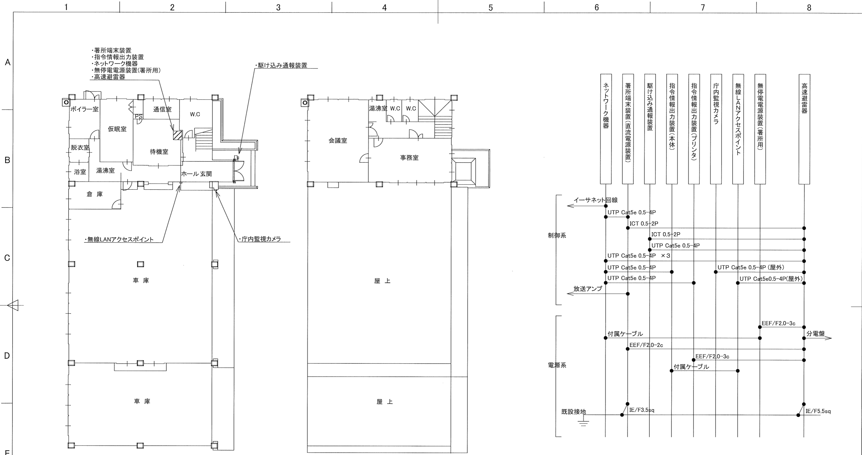
1階 平面図
